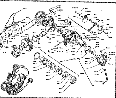
2 e Groupe Coque Planche 1
